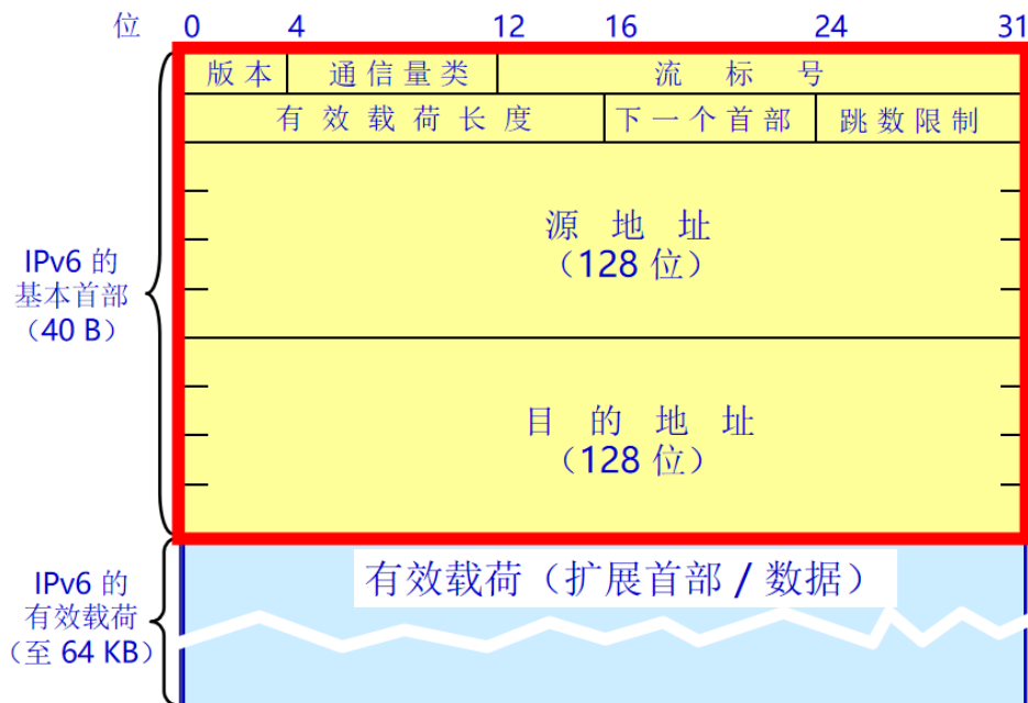
40 字节长的 IPv6 基本首部
