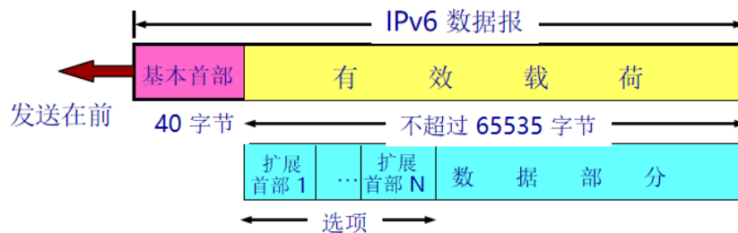
具有多个可选扩展首部的 IPv6 数据报的一般形式
